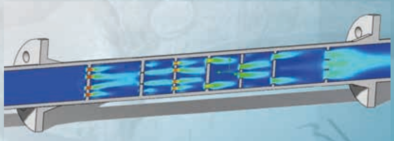
Скорость потока с многоотверстной диафрагмой
